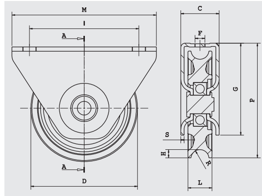
Yarım daire kanallı, dıştan taşıma plakalı tek sıra rulmanlı çelik tekerlek.
